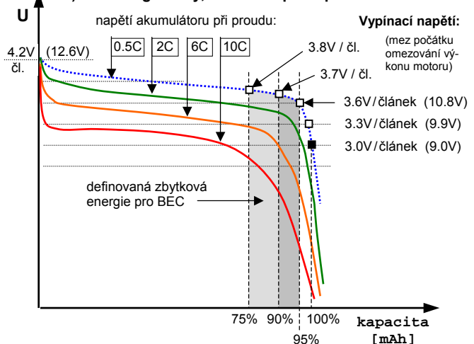
b) TMM® regulátory, nastavení pro Lipol baterie
