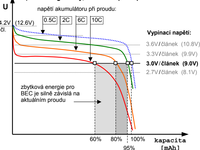
a) běžné regulátory, nastavení pro Lipol baterie
